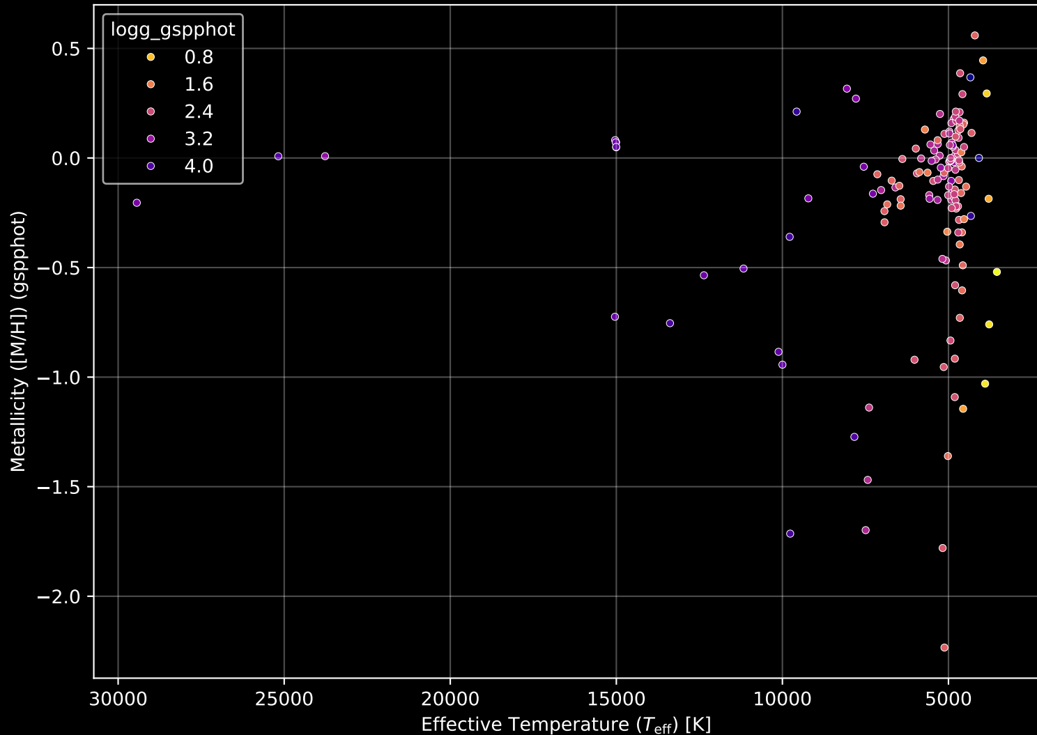
APOGEE DR17 Field: [Lac_3] Stellar Population Parameters (n= 147)
